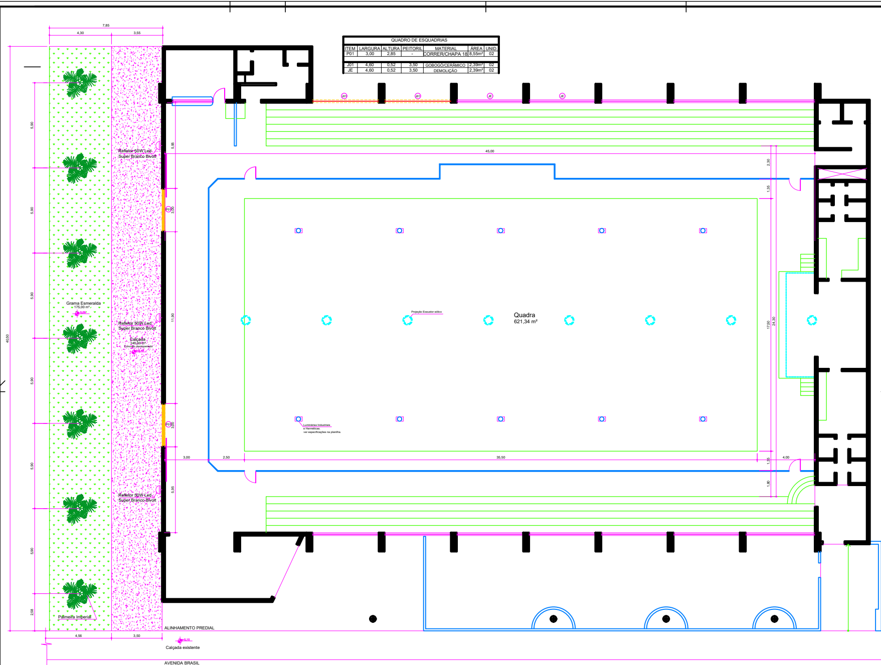
PLANTA BAIXA GINÁSIO DE ESPORTES ESC. 1:100
